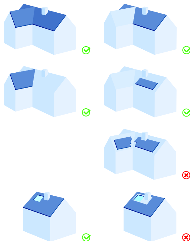
Abb. 13 Aussparungen schliessen
